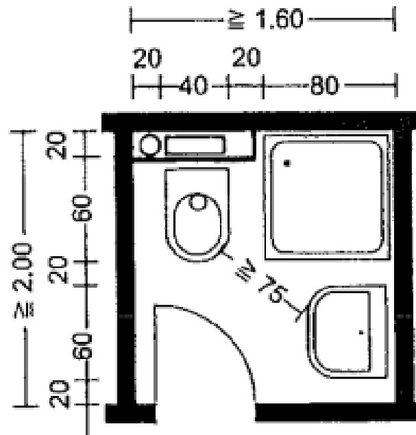
2 pav. Vonios kambario įrangos išdėstymo mažose patalpose pavyzdys.
